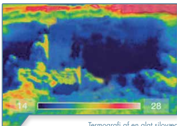
Termografi af en glat silovæg
